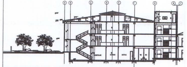
A-A KESİTİ ölçek:1/100
